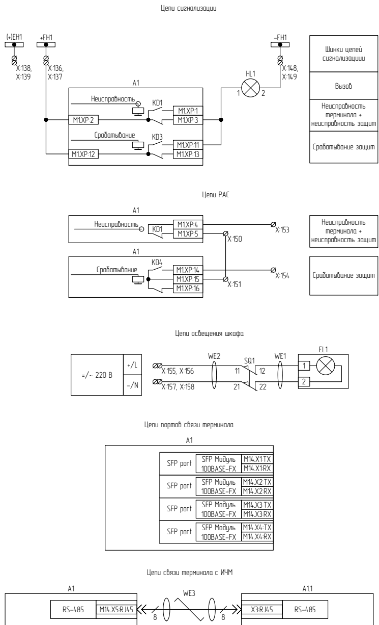
Рисунок В.3 – Схема электрическая принципиальная (часть 3)
